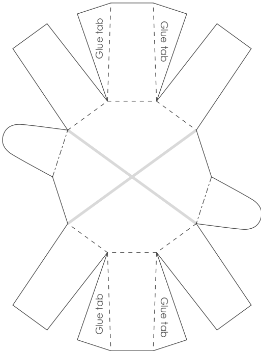
False bottom
